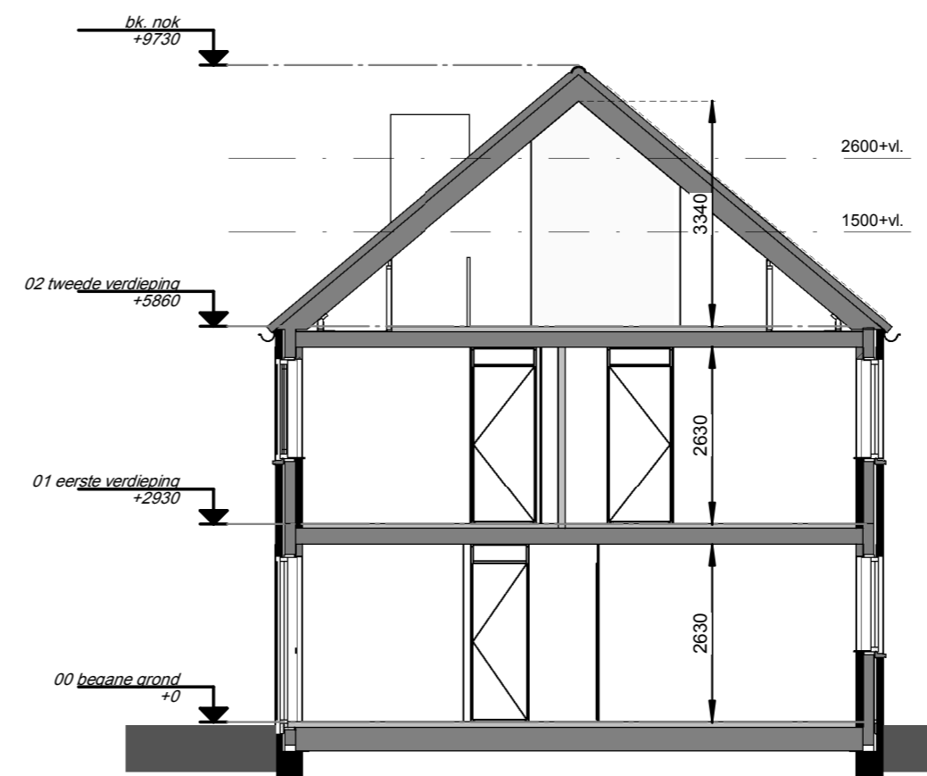
Doorsnede
