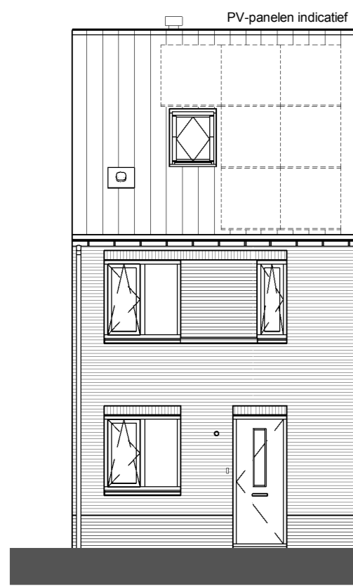
Voorgevel
