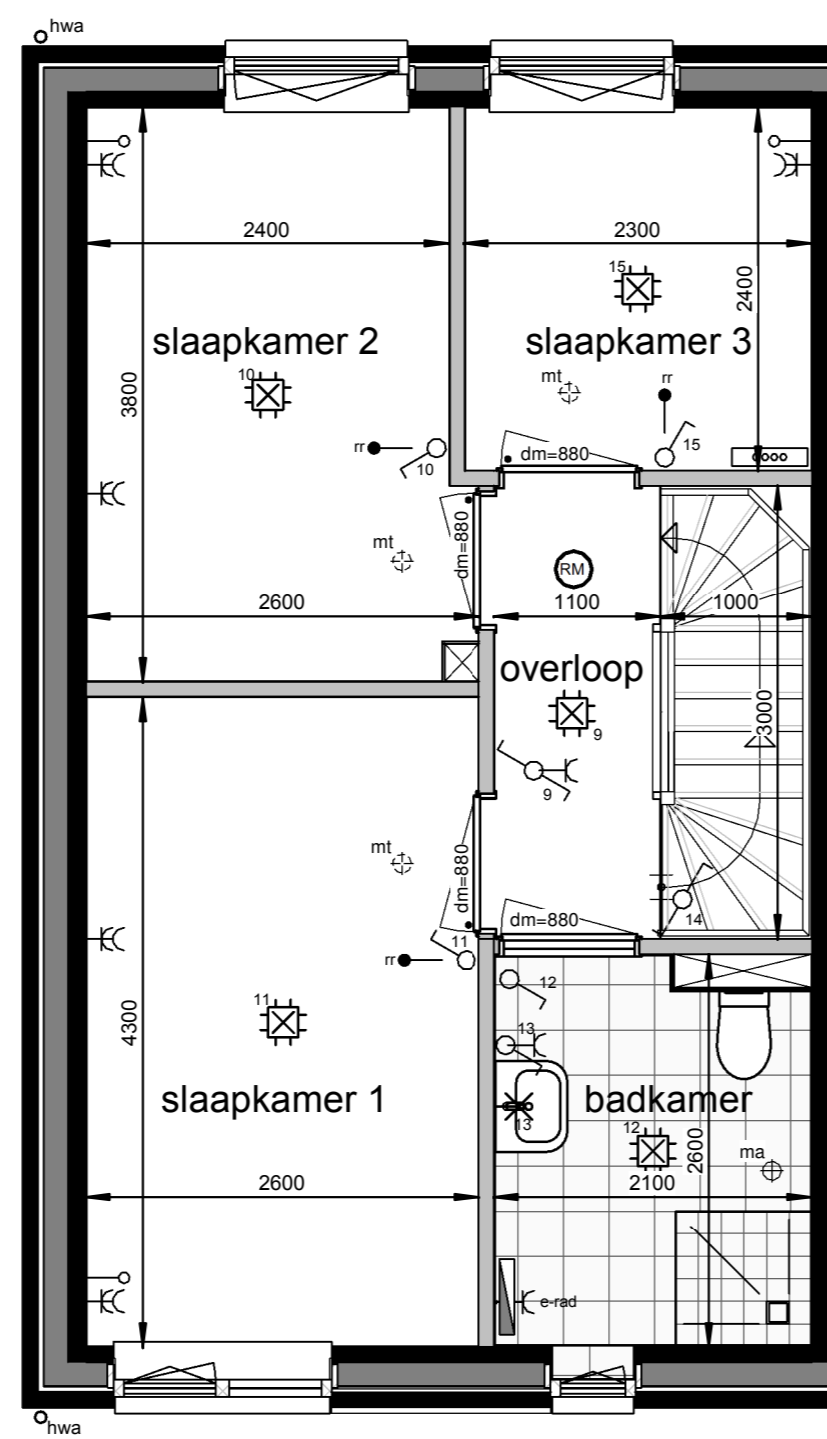
Eerste verdieping
